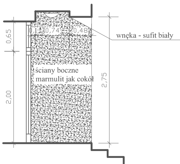
Wnęka wejściowa przekrój skala 1:50
